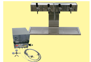
Durchlaufkühler mit Schanksäule 4-leitig, Clean-Ball und CO 2 Schlüssel/Flow cooler with 4-sided dispensing column, clean ball and CO 2 key (0019) € 545,00
