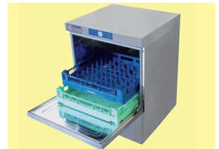
Geschirrpülmaschine, gewerbl., Wechselkorb-Version, 2-4 Min.-Programm/Professional dishwasher, interchangeable basket-system, 2-4 min. program 230 oder 400 V, 7,5 kW, 60 x 82,5 x 60 cm
